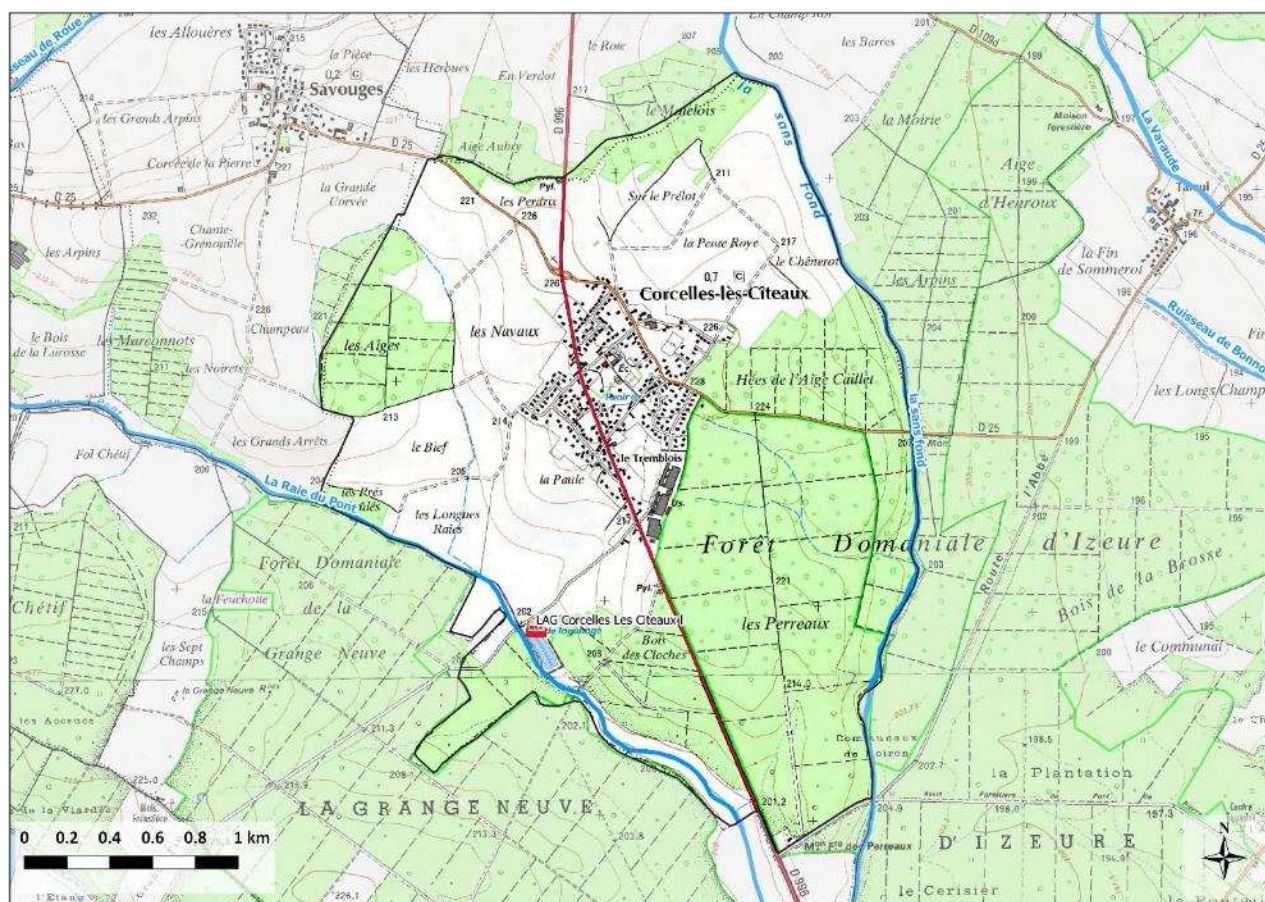
Réseau hydrographique de la commune de Corcelles-lès-Cîteaux
