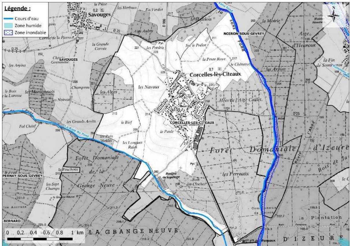
Zones humides et inondables recensées sur la commune de Corcelles-lès-Cîteaux
