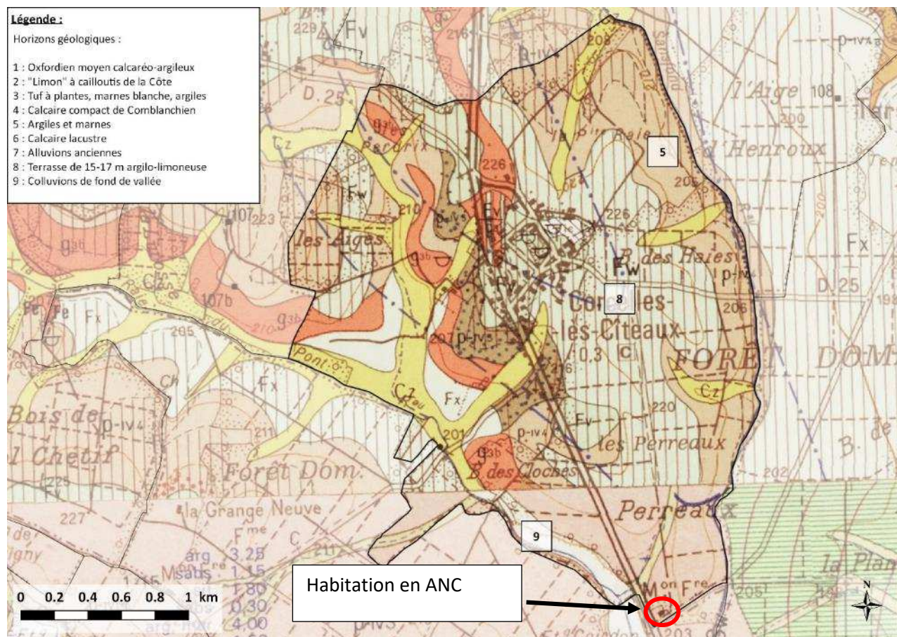
Analyse du milieu physique
